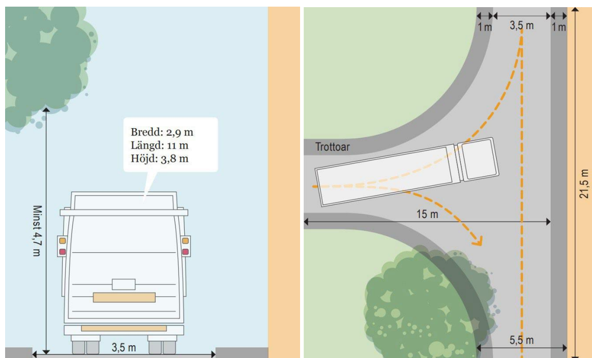
Figur 1. Transportvägens mått och vändplats i trevägskorsning (Avfall Sverige, 2023).
