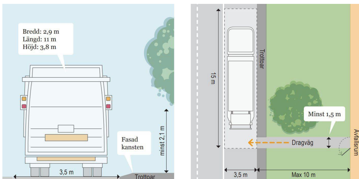
Figur 3. Dragvägens utformning (Avfall Sverige, 2023).
