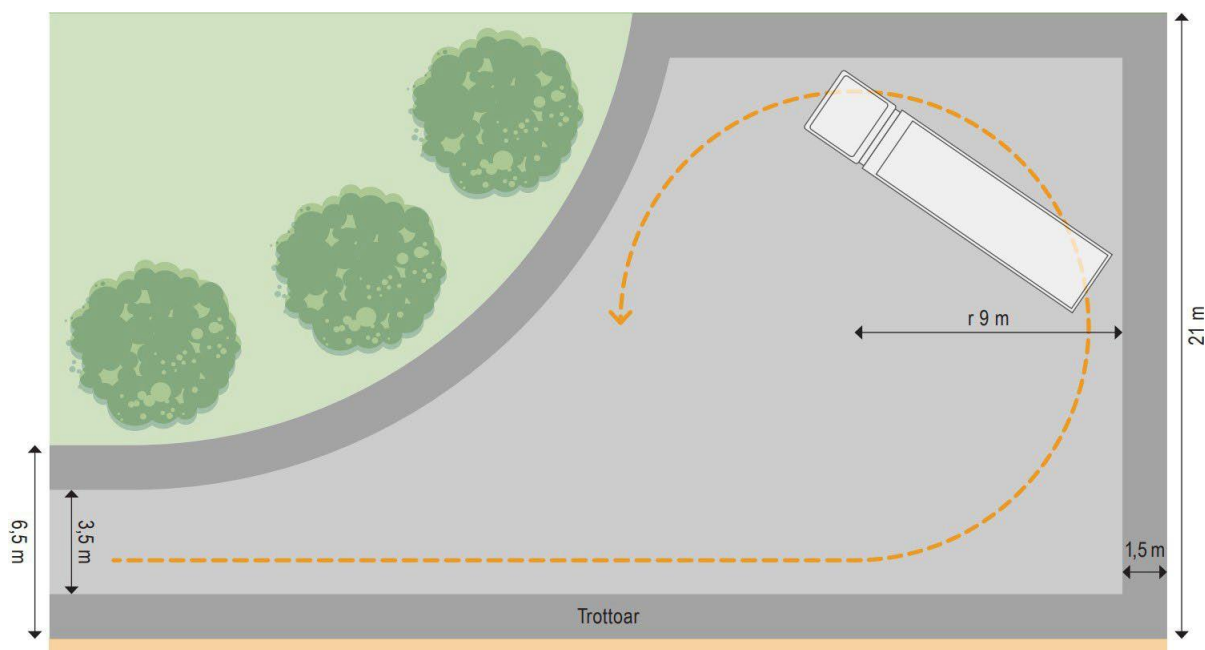
Figur 2. Vändplatsens mått (Avfall Sverige, 2023).
